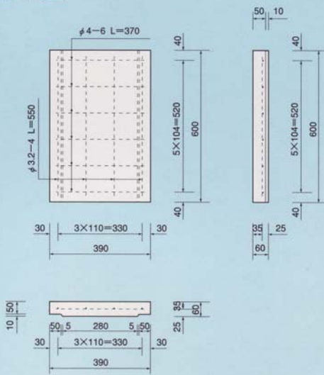
歩道用甲蓋
