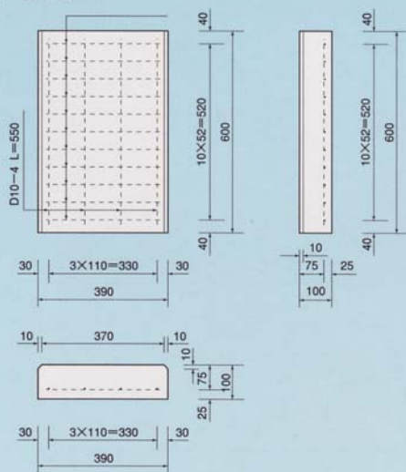
甲蓋（普通型）
