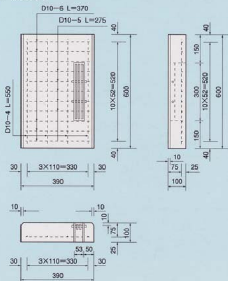
甲蓋（網付）
